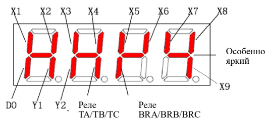
Рис. 6-28 Схема отображения текущего состояния статусов клемм
