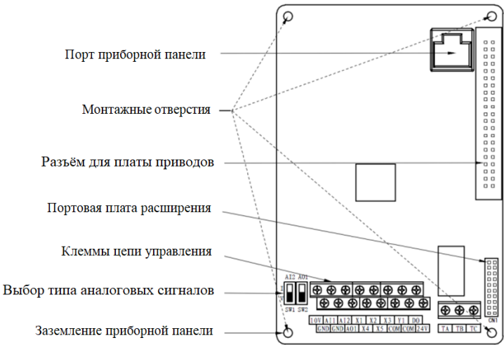
Рис. 3-16 Плата управления
