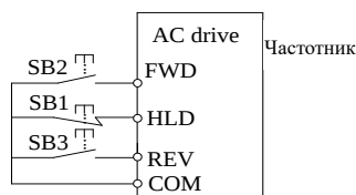
Рис.6-15 Трехпроводной режим управления 1
