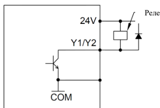
Рис. 3-12 Способ подключения внутреннего источника питания +24 В
