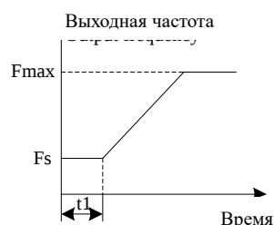
Рис.6-3 Пусковая частота и время выдержки пусковой частоты
