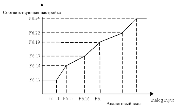
Рис. 6-17 Нелинейная кривая аналогового входа
