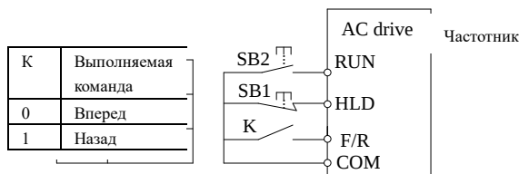
Рис.6-16 Трехпроводной режим управления 2
